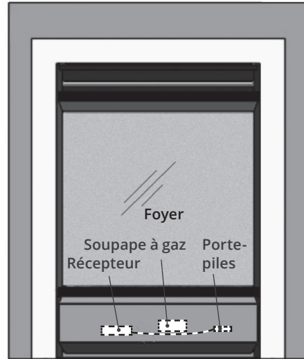
Porte-piles situé à côté de la soupape sous la boîte de foyer derrière le panneau d'accès.
